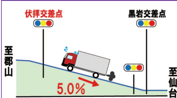
一般国道4号断面図
